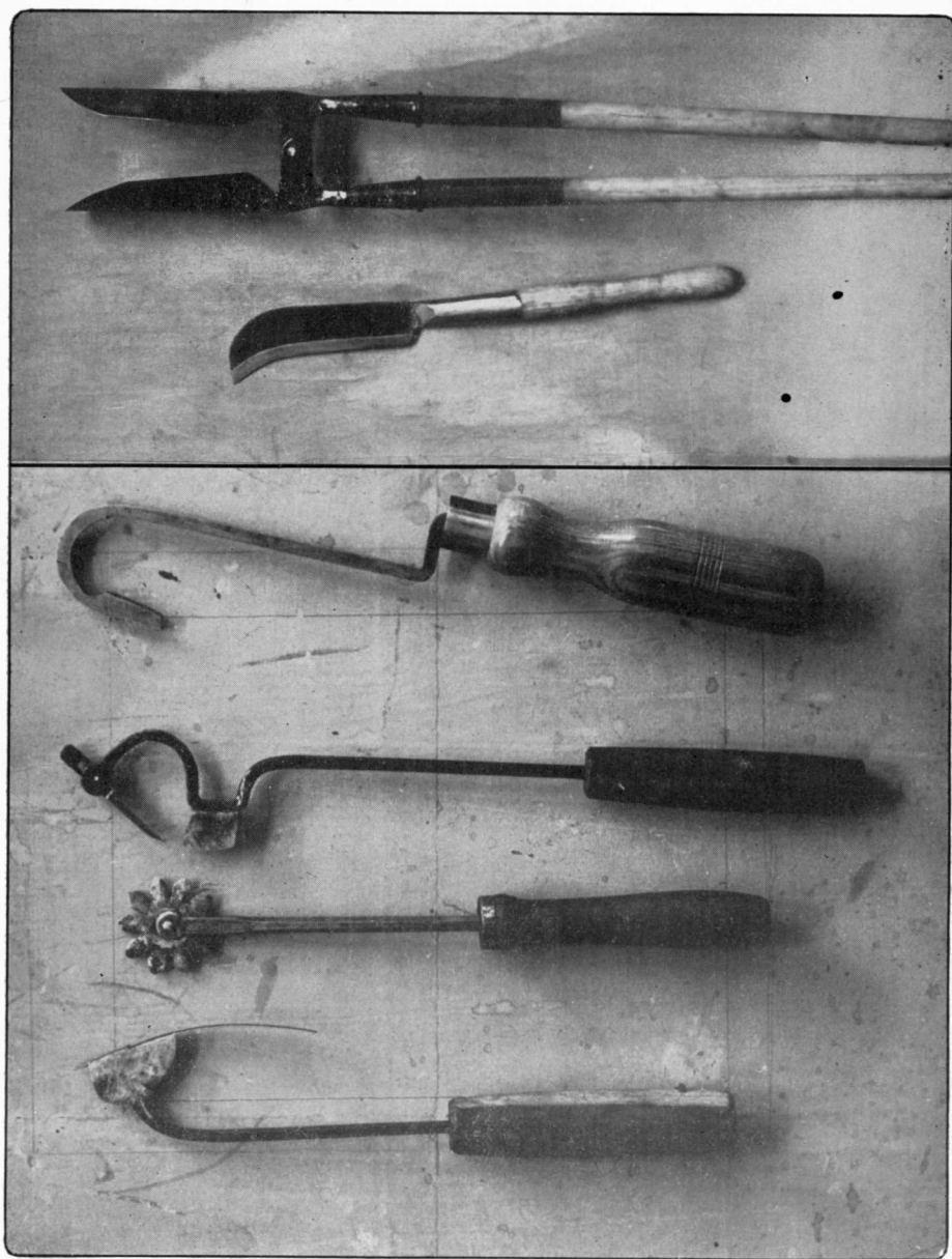
PLATE XV (a).—PODÃO OU MACHETE, E PAR DE PÁS EM THESOURA PARA A TRANSPLANTAÇÃO DE FLANTAS NOVAS.
